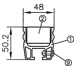
Bundschraube
