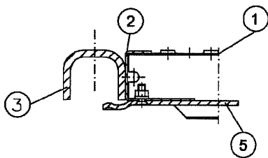
Schnitt Auflagerklaue
