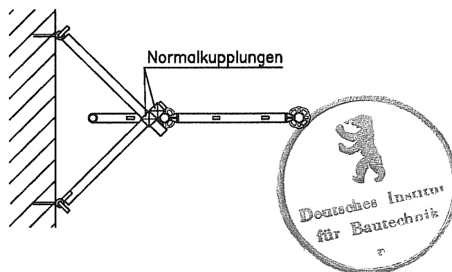
Bild C.2c: V-Halter
