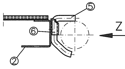
Schnitt B-B
