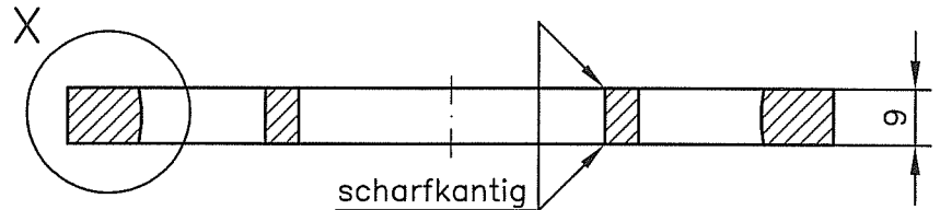
Schnitt A-B
