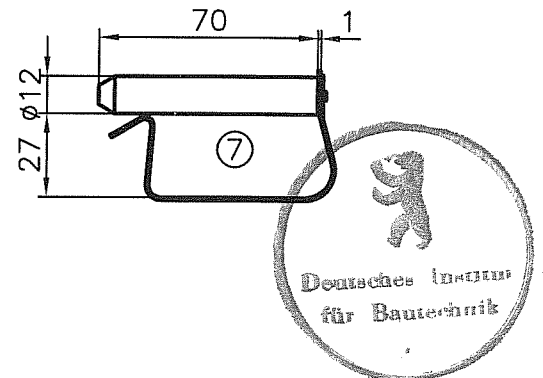
Federsteckbolzen KSB55
