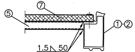
Schnitt B-B
