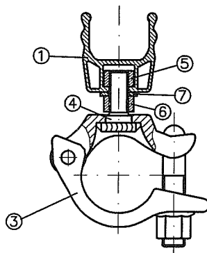
Bundschraube
