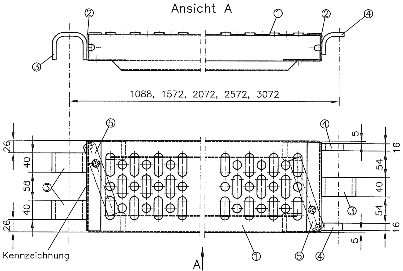
Schnitt Auflagerklaue
