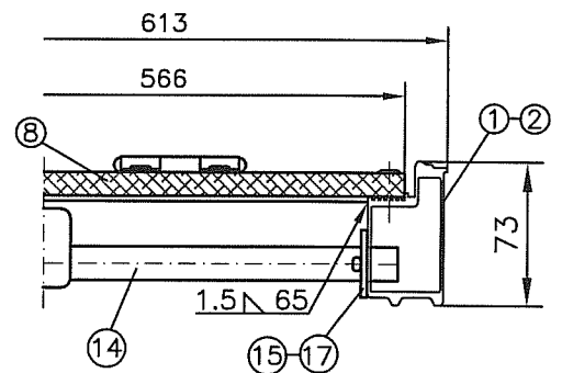
Schnitt B-B
