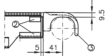
Schnitt A-A
