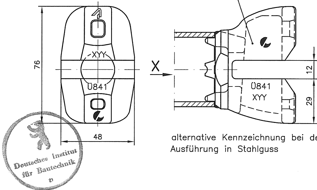
Ansicht X
