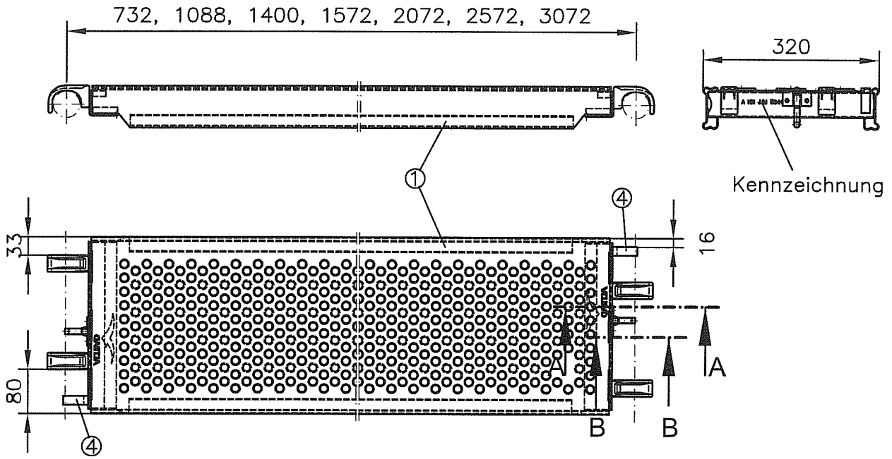
Ansicht Z
