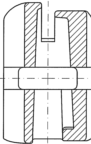
Schnitt A-B
