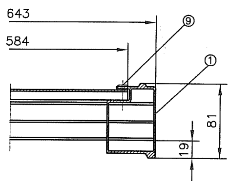
Schnitt A-A
