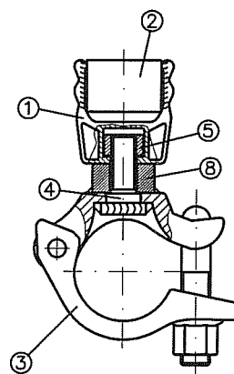
Ansicht A
