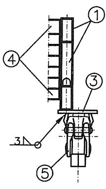
Ansicht W
