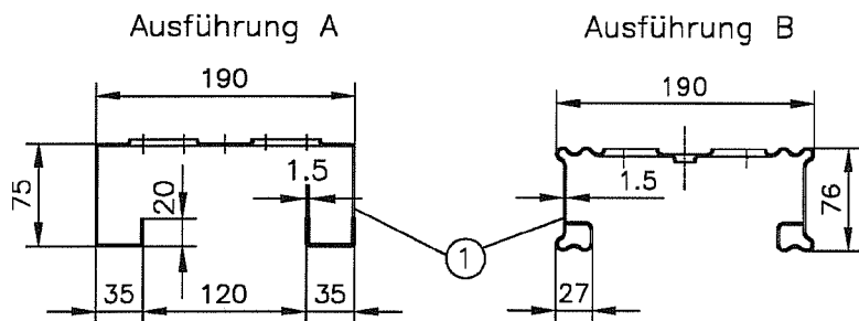
Querschnitt
