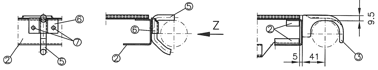
Ansicht Z
