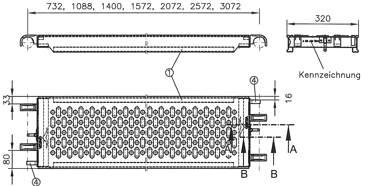
Ansicht Z
