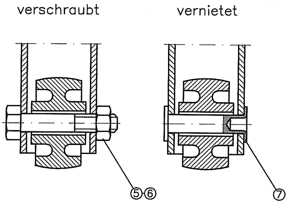
Schnitt A-A Rolle Pos. 4
