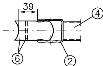
Ansicht A
