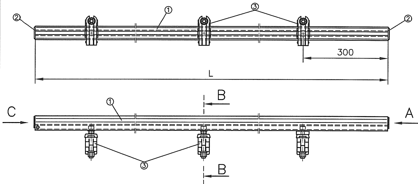
Ansicht C
