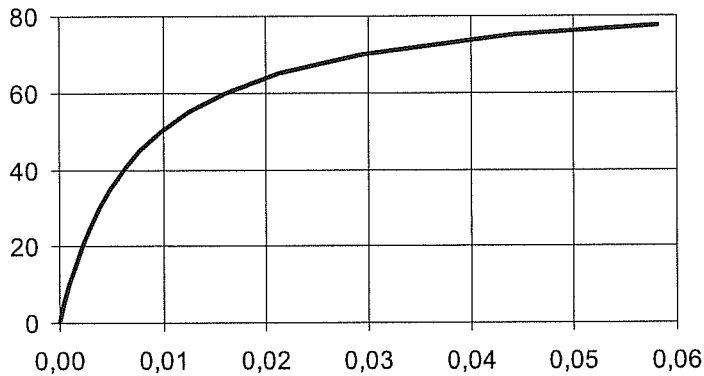
Bild 1: Drehfedersteifigkeit im Riegelanschluss der "Version I" in der vertikalen Ebene
