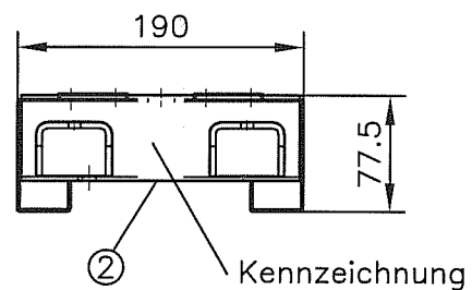
Kopfbeschlag
