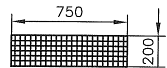
Gitterrost (P Pressrost)
