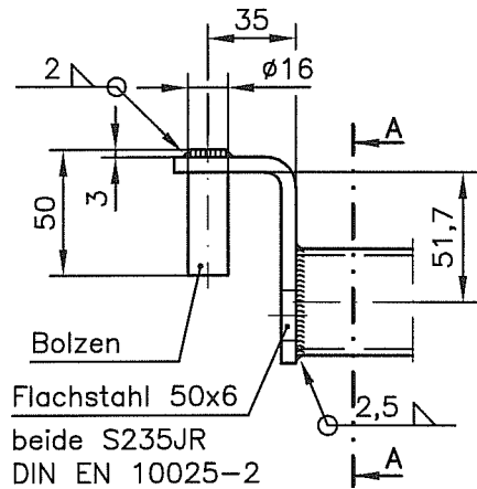
Ansicht W
